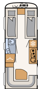
510 ER 4 sovepladser
